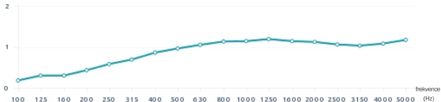
Vážený součinitel zvukové pohltivosti ( \alpha_w )
